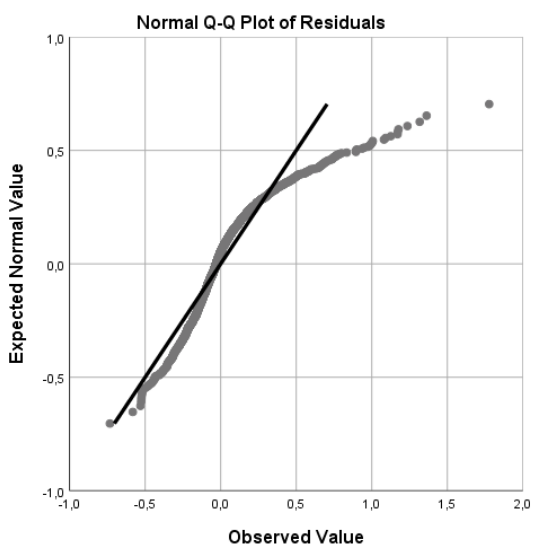
Figuur 8: Q-Q plot van de residuen
