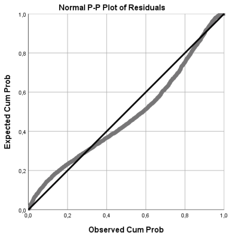
Figuur 11: PP-plot met residuen van de getransformeerde afhankelijke variabele
